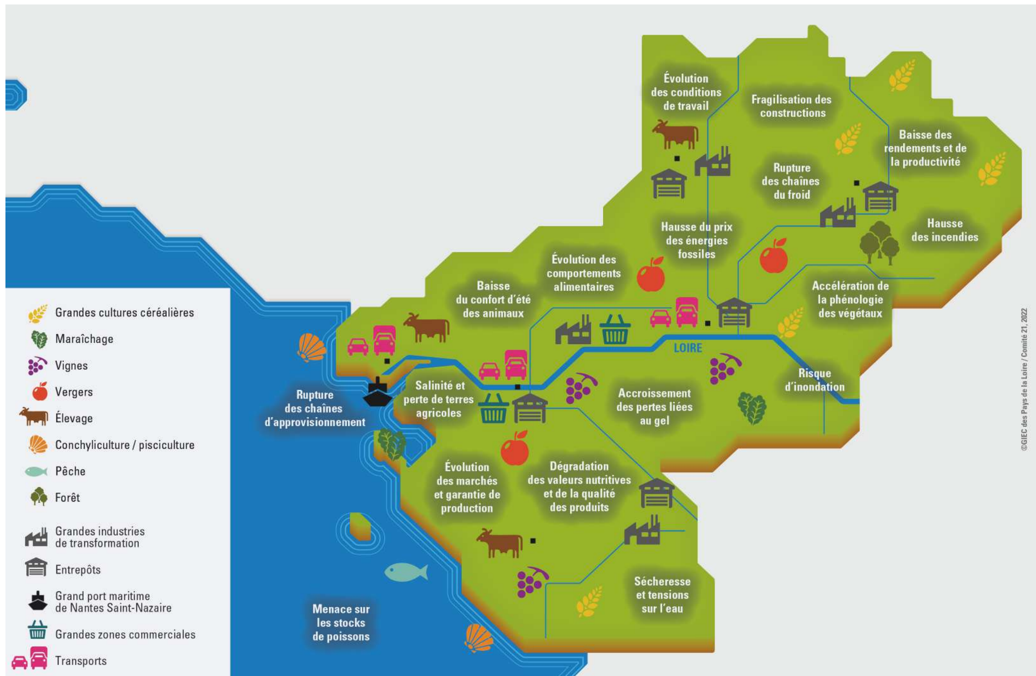
FIG. 26 • VULNÉRABILITÉS DU SYSTÈME ALIMENTAIRE FACE AUX CHANGEMENTS CLIMATIQUES
