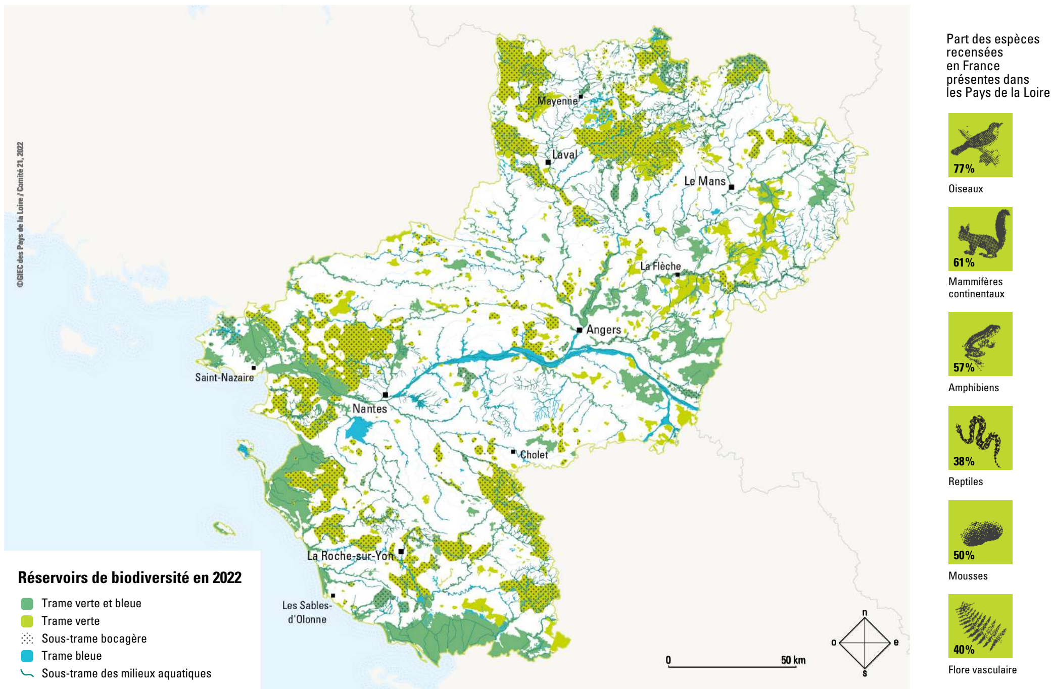
FIG. 2 • RÉSERVOIRS DE BIODIVERSITÉ DANS LES PAYS DE LA LOIRE
