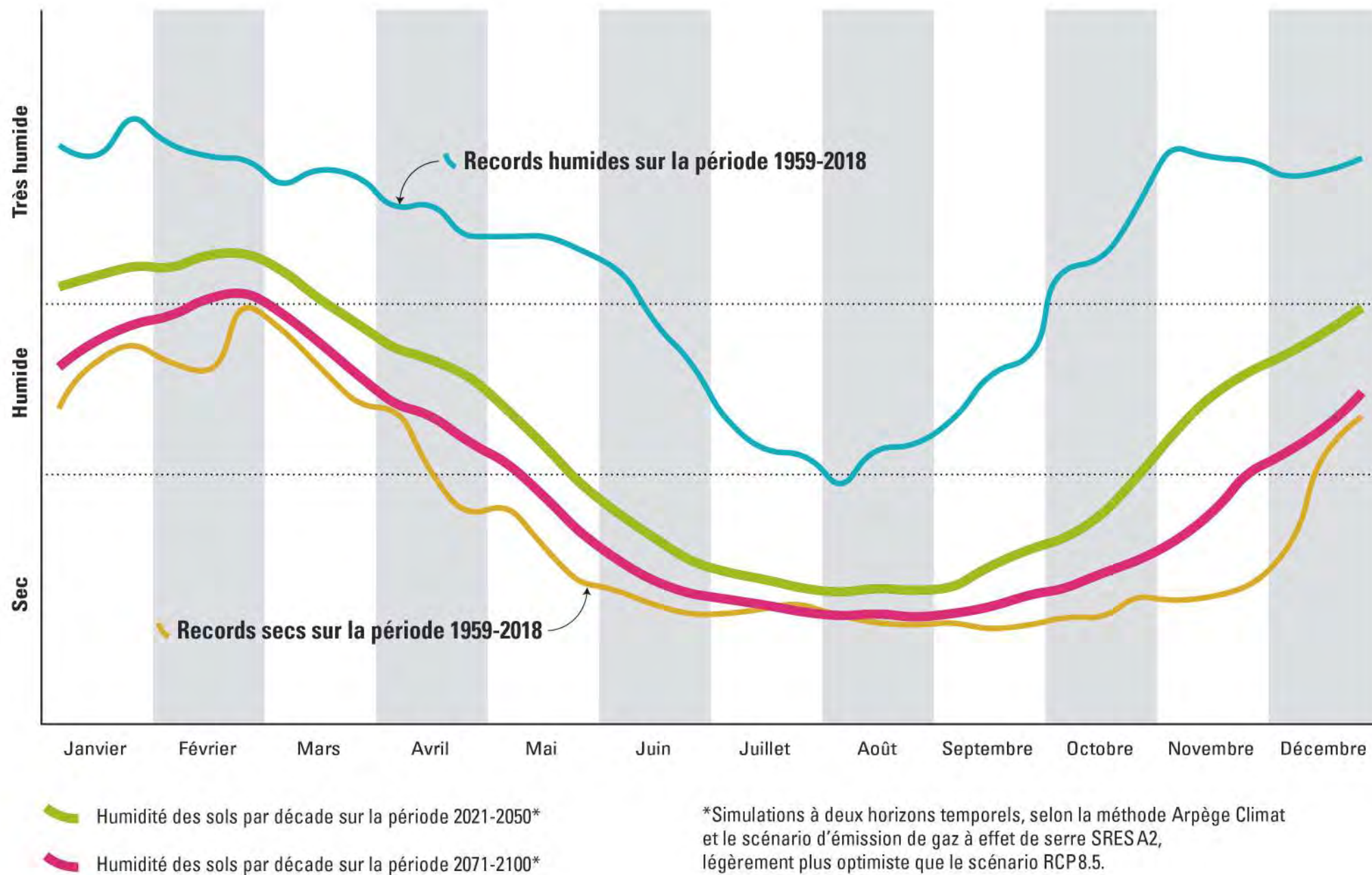
FIG. 15 • ÉVOLUTION DE L'HUMIDITÉ DES SOLS
